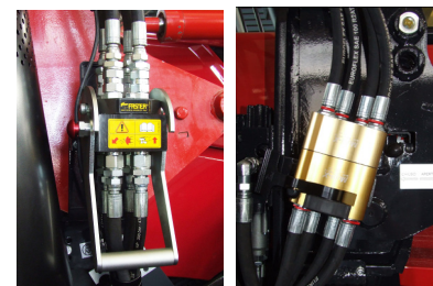
Innesto rapido multiplo FASTER OPTIONAL Innesto rapido multiplo CEJN OPTIONAL Multi-connector device FASTER OPTIONAL Multi-connector device CEJN OPTIONAL
